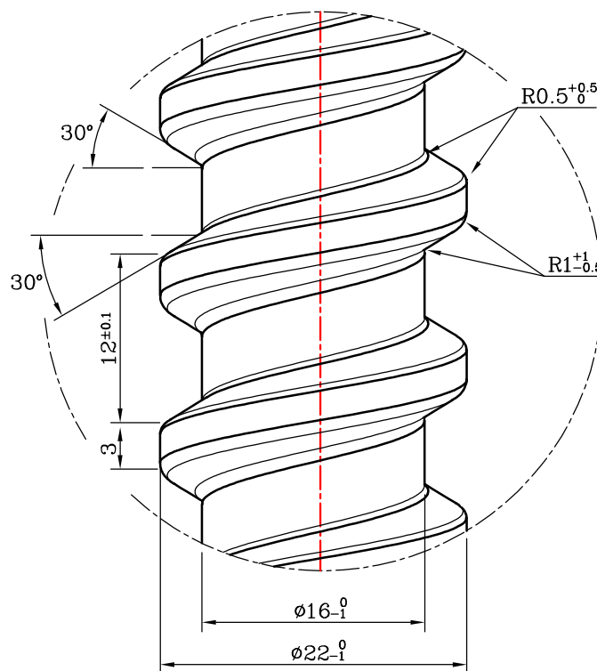
DETAIL Scale: 3
